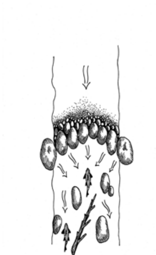
Figur 14. Ett klassiskt exempel på hur konstgjorda forsnackar skapats i form av en tröskel. Detta genererar en hölja nedströms. Trösklar av detta slag ska slutta svagt in mot mitten. De bör förstärkas/tätas med mindre sten och grus. Genom att vinkla med spetsen uppströms erhålls vattenströmmar in mot mitten, varvid erosion av kanter motverkas. Observera att naturliga trösklar inte är så här ingenjörssitade (jämför Figur 6). Sträva efter ett mer naturligt utseende.
