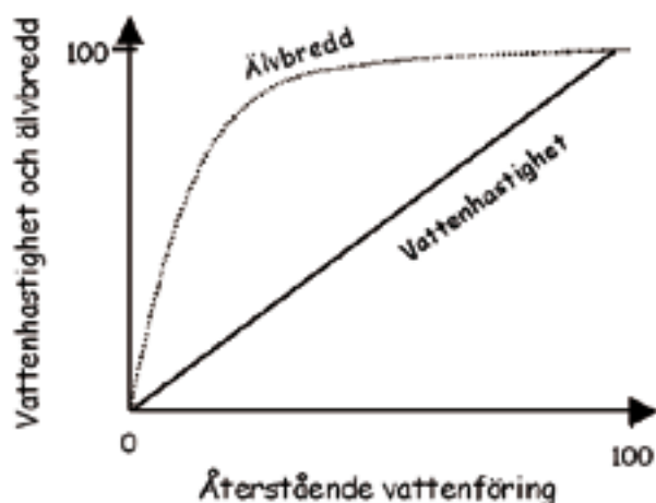
Figur 3. Samband mellan vattenföring (från 0–100 % av naturligt flöde) och medelvattenhastighet resp vattendrags bredd. Figur: Ingemar Näslund, Länsstyrelsen i Jämtlands län.
