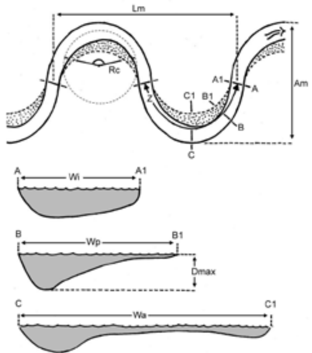
Figur 11. En idealiserad bild av ett meanderande vattendrag. Bilden är inte med som ett förslag på lösning utan för att få en gemensam terminologi.
