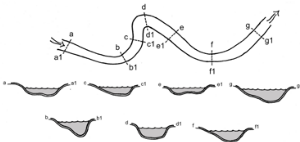
Figur 12. Ett typiskt meanderande vattendrag med de naturliga djupförhållandena i olika avsnitt. Jämför med Figur 11. Ofta gräver man inte djupförhållandena på detta sätt, det blir för kostsamt. Bättre är att eftersträva en enklare fåra men med grundmönstret, t.ex. thalwegens position, markerad. Vattendraget får sedan själv mejsla fram det slutliga utseendet.
